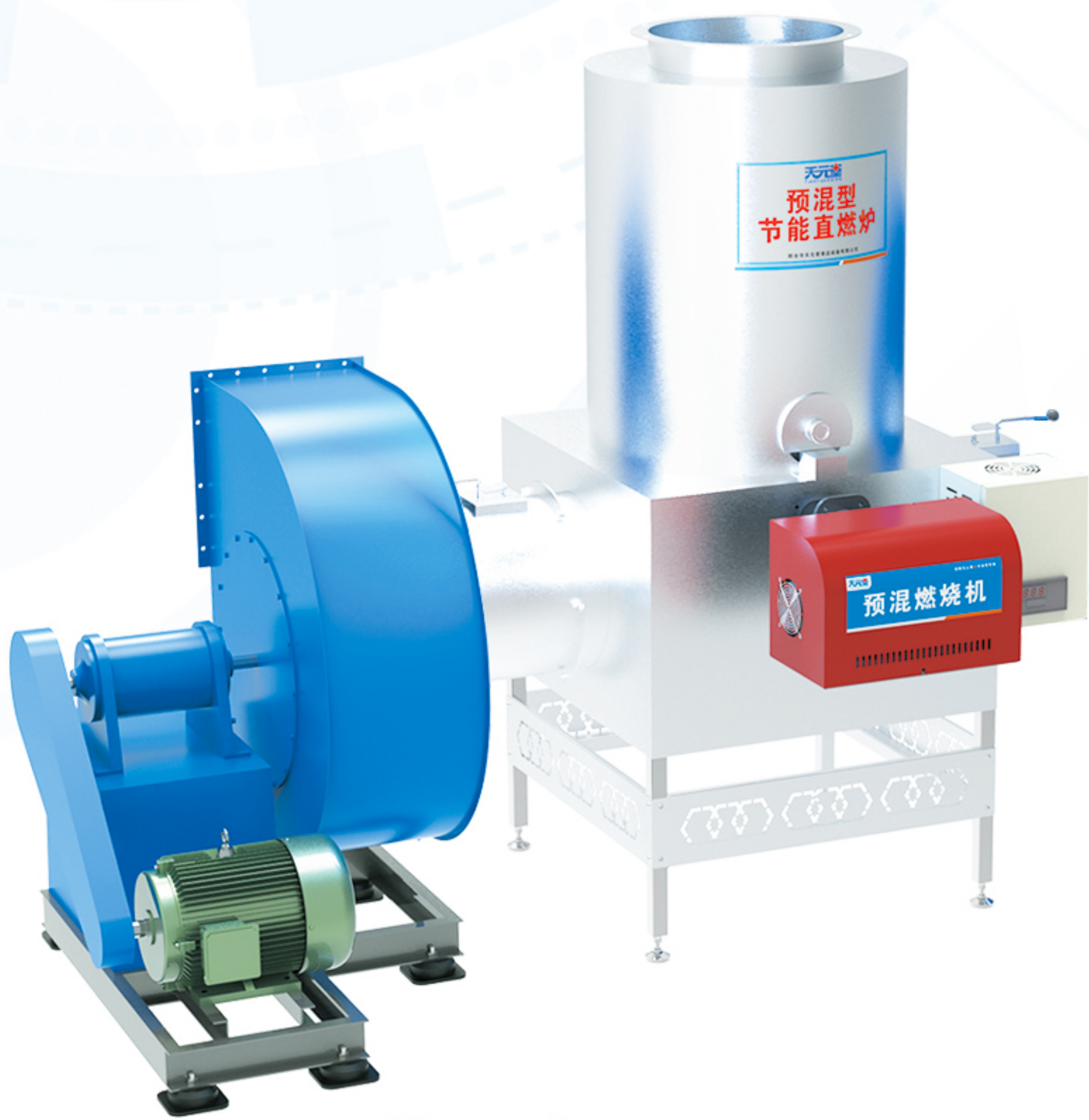
带一台风机图示
